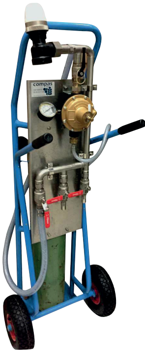
CHARIOT INERTAGE MOBILE 1 à 3 VOIES
